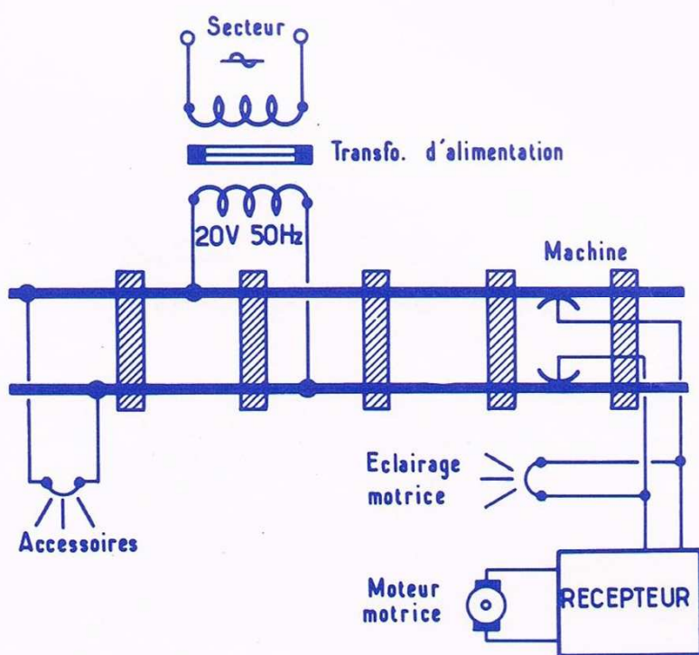
Fig. 1. — Alimentation du réseau miniature.
