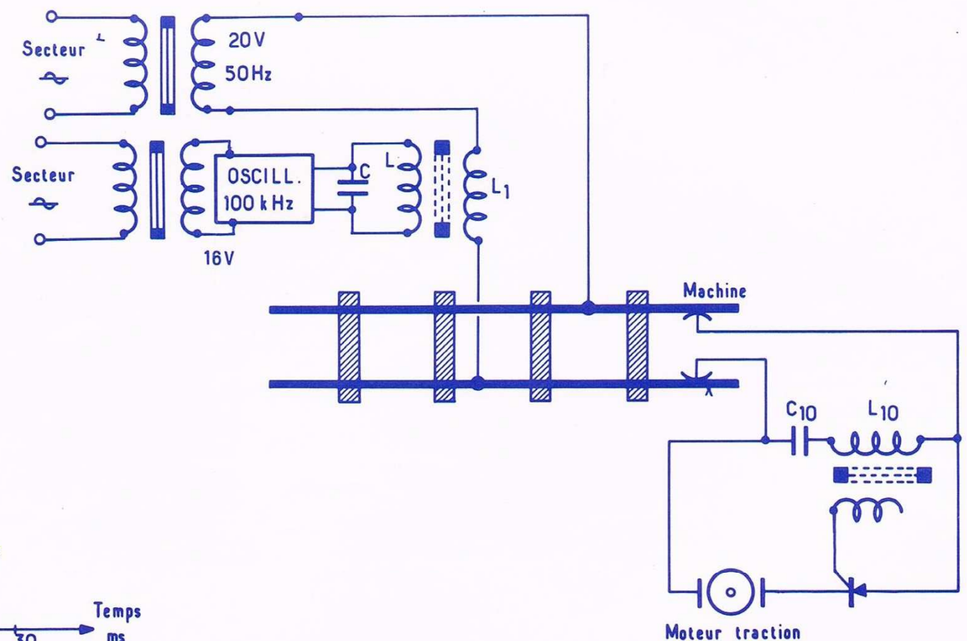
Fig. 2. — Mise en place de l'émetteur ultrasonore.
